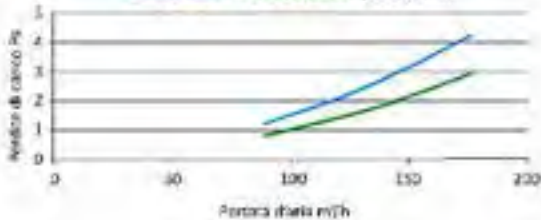
Curva a 90° - Curva a 45° Ø160 mm
